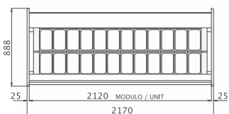
Lunghezze moduli per tutte le versioni
